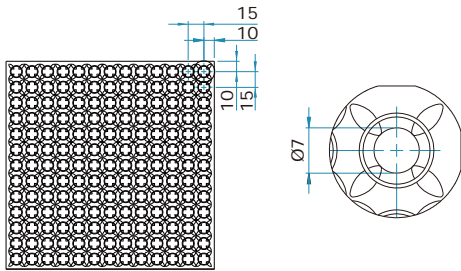
optical panel(OP-100-01)/front
