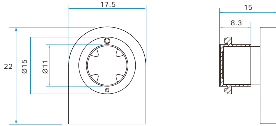
optical panel(OP-100-01)/front
